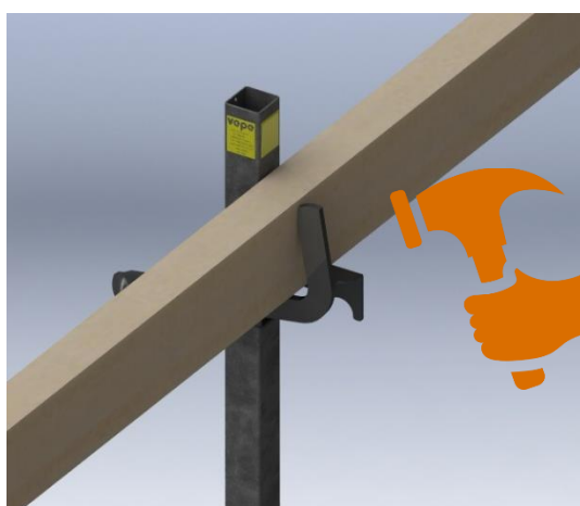
Kiristä lukot kunnolla vasaralla lyöden
