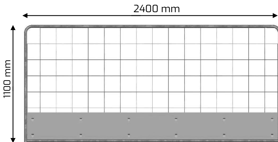
Turvakaiteen verkkoelementti
